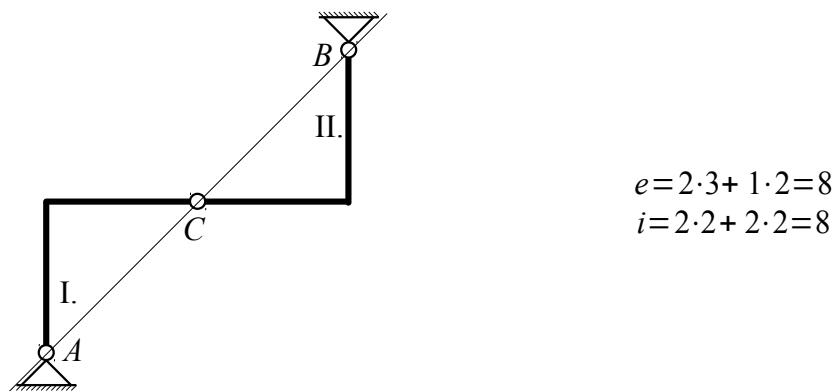
B5.4. ábra. Statikailag határozatlan és túlhatározott összetett szerkezetek
