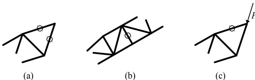
B6.9. ábra. Speciális csomópontok vakrudakkal
