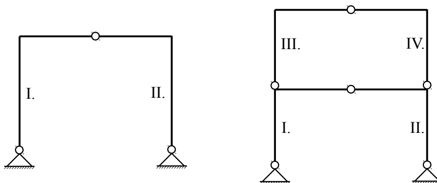
B3.3. ábra. Összetett keretszerkezetek
