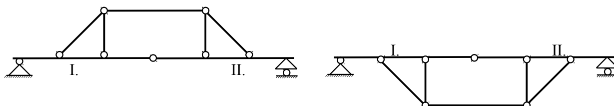
B3.4. ábra. Függesztőműves (bal oldali ábra) és feszítőműves (jobb oldali ábra) tartó
