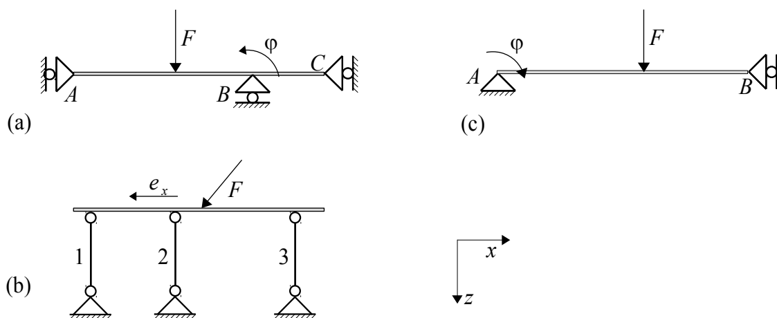
B2.2. ábra. Statikailag túlhatározott szerkezetek ( i=3 )
