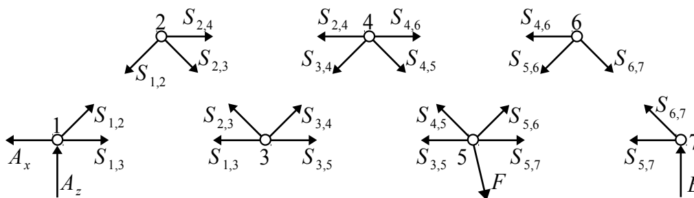
B6.2. ábra. A csomópontján terhelt rácsos tartó elkülönített csomópontjai
