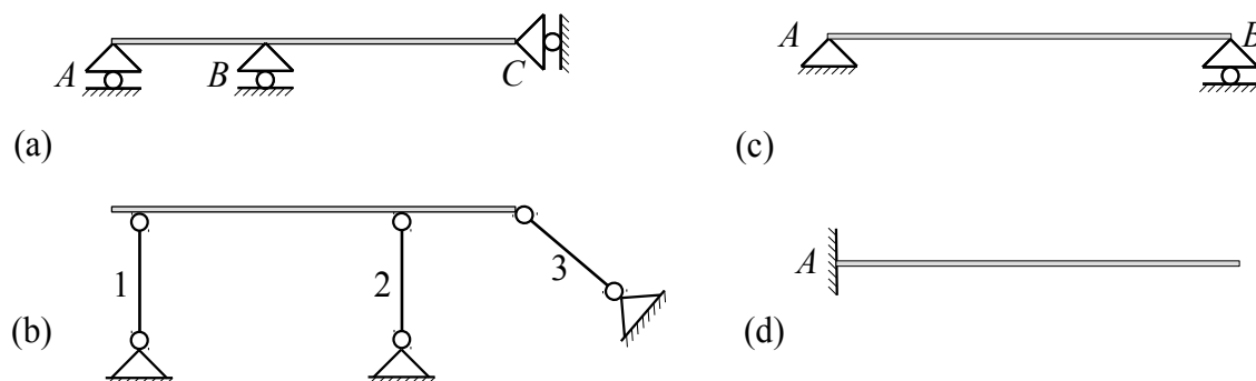
B2.1. ábra. Statikailag határozott egyszerű tartók
