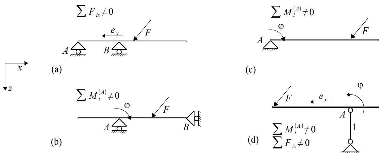
B2.3. ábra. Statikailag túlhatározott szerkezetek ( i < 3 )
