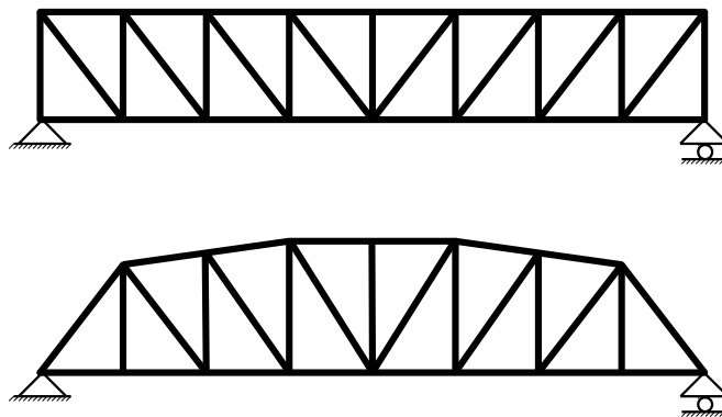
B6.5. ábra. Oszlopos vagy Pratt-féle rácsozású rácsos tartók.
