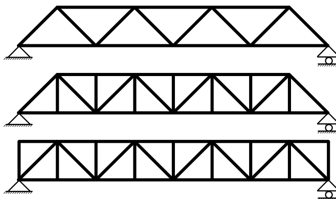
B6.4. ábra. Szimmetrikus vagy Warren-féle rácsozású rácsos tartók
