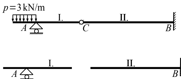
B4.2. ábra. Gerber-tartó (felső ábra) és a tartó fix (II.), illetve befüggesztett (I.) része külön ábrázolva, saját külső kényszereikkel (alsó ábra)
