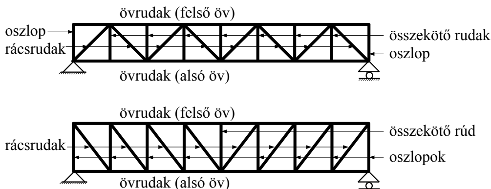
B6.3. ábra. A különböző helyzetű rudak elnevezése
