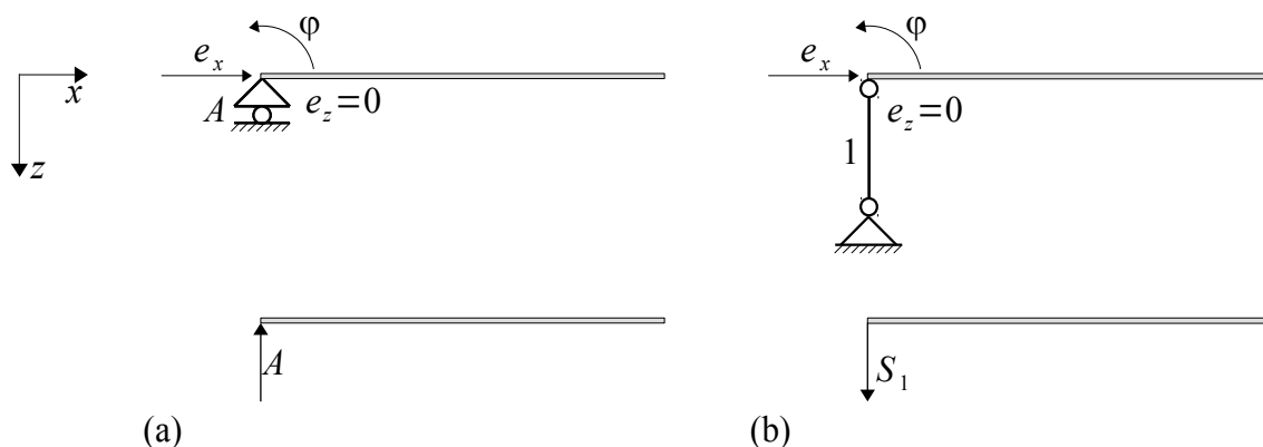
B1.1. ábra. Megtámasztás görgővel (a) és rúddal (b)
