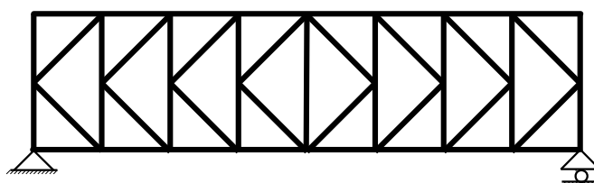
B6.6. ábra. K-rácsozású tartó
