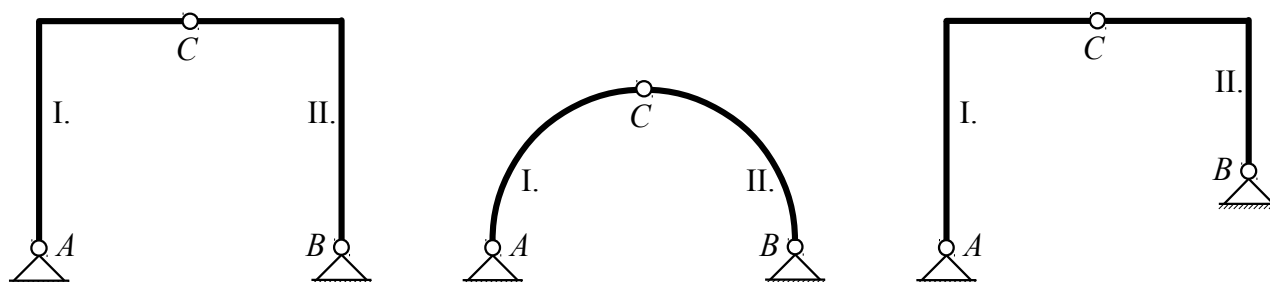
B5.1. ábra. Háromcsuklós tartók
