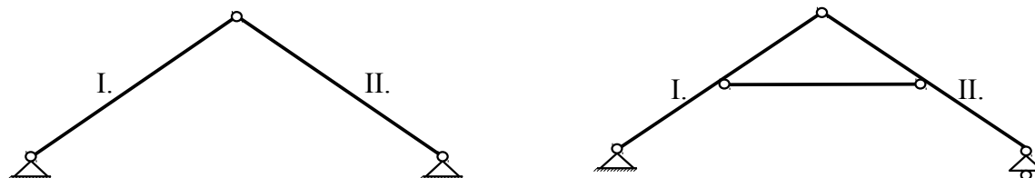
B3.1. ábra. Fedélszékek statikai modelljei, üres fedélszék (bal oldali ábra) és fogópárral merevített fedélszék (jobb oldali ábra)
