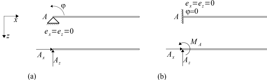
B1.2. ábra. Csuklós megtámasztás (a) és befogás (b)
