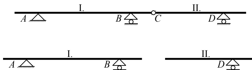
B4.1. ábra. Gerber-tartó (felső ábra) és a tartó fix (I.), illetve befüggesztett (II.) része külön ábrázolva, saját külső kényszereikkel (alsó ábra)
