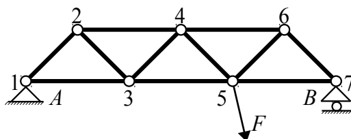
B6.1. ábra. Csomópontján terhelt rácsos tartó
