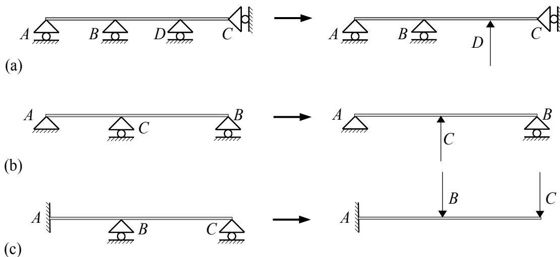
B2.4. ábra. Statikailag határozatlan szerkezetek ( i > 3 )
