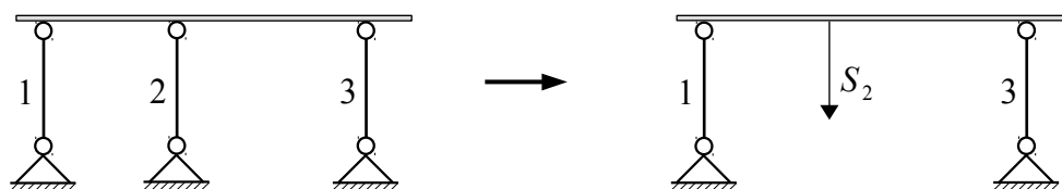
B2.5. ábra. Statikailag határozatlan szerkezet ( i=3 )
