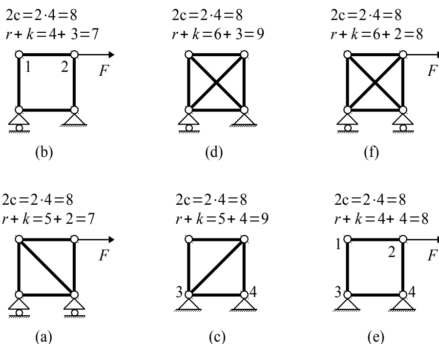
B7.1. ábra. Statikailag túlhatározott (a,b), statikailag határozatlan (c,d) és egyidejűleg statikailag határozatlan és statikailag túlhatározott (e,f) rácsos szerkezetek
