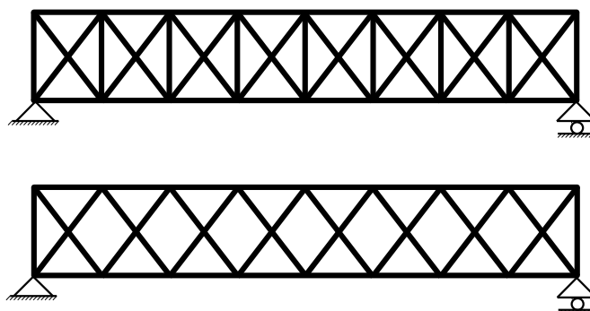
B6.7. ábra. X-rácsozású tartók
