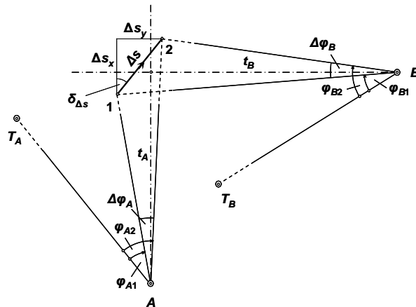
5-2. ábra. Vízszintes elmozdulásmérés szögváltozások mérésével
