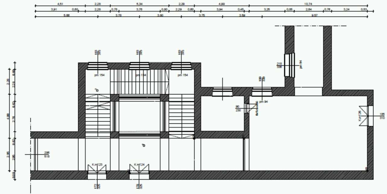
1. emelet alaprajzi részlete m = 1:100
